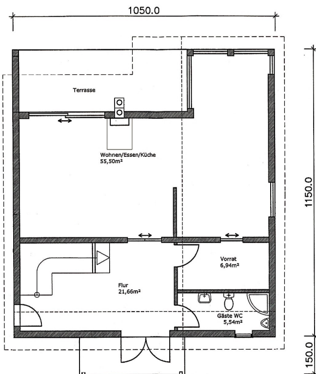
ERDGESCHOSS
