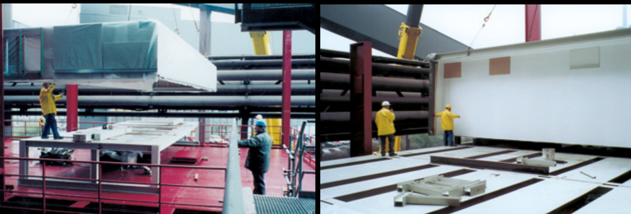
Schalhausmontage auf einer 6-Meter-Bühne in Duisburg-Nord.
