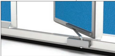
Türschließer (Panel unten)
