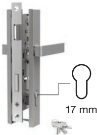
Euro-Zylinderschloss Zylinder 30/35 mit 3 Schlüsseln
