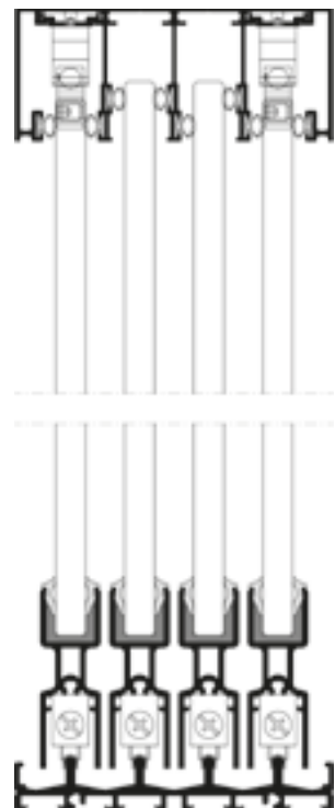
heroal S 20 C, Schnittdarstellung
