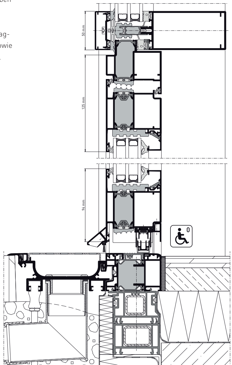
heroal D 72, Schnittdarstellung Fassadenintegration
