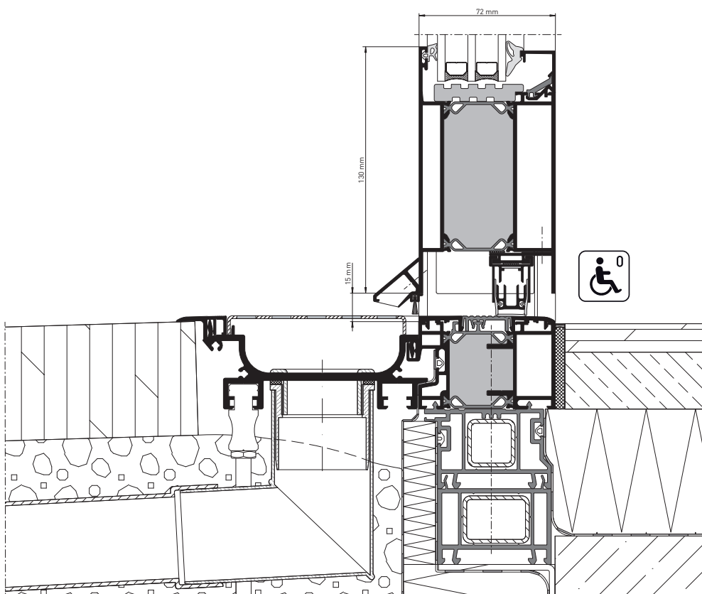
heroal D 72, Schnittdarstellung Null-Barriere nach DIN 18040
