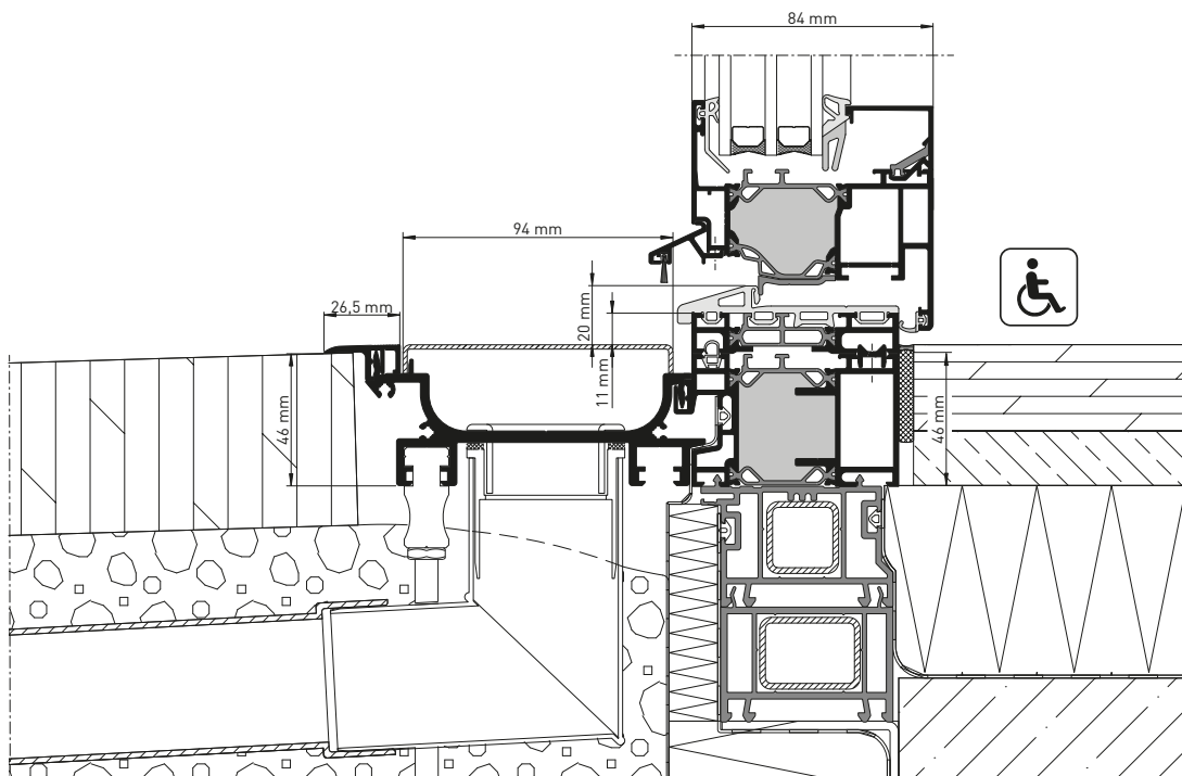
heroal W 72 mit heroal DS, Schnittdarstellung
