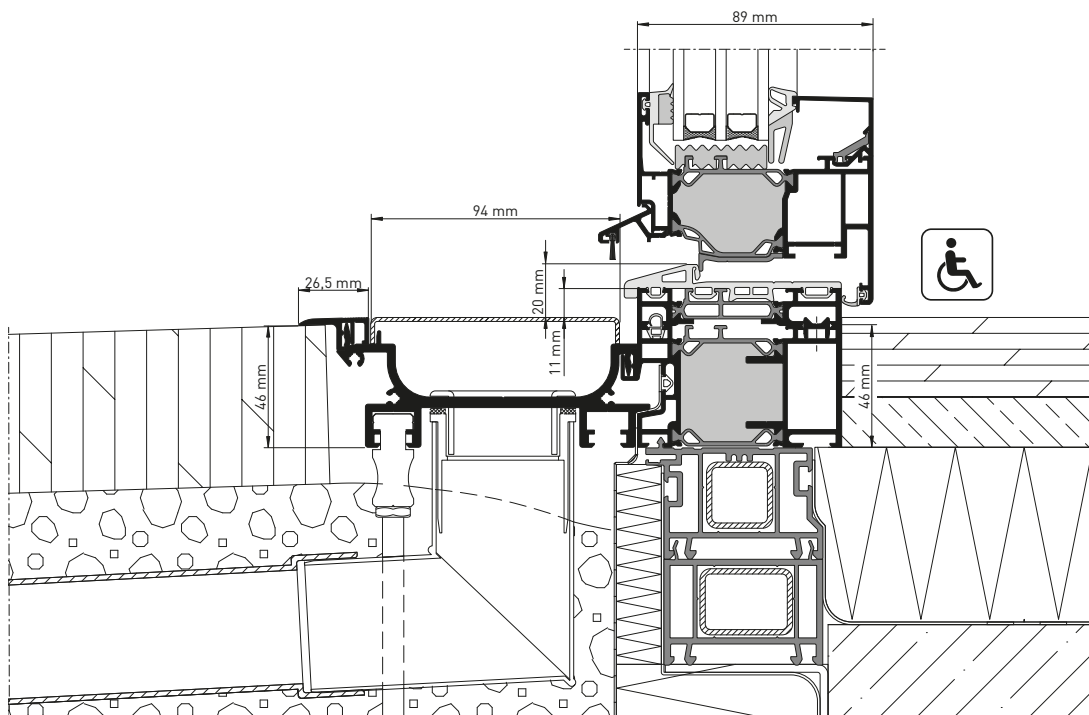
heroyal W 77 mit heroyal DS, Schnittdarstellung
