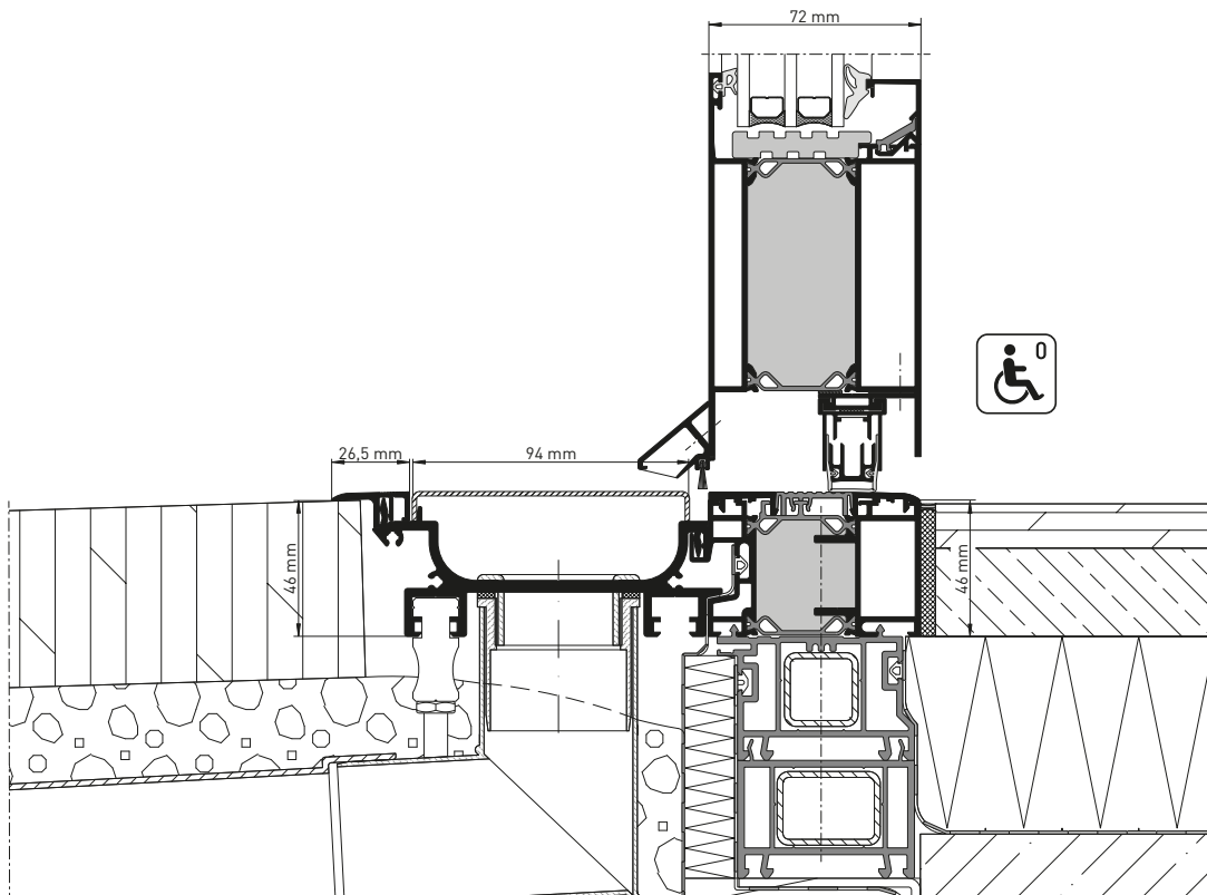
heroal D 72 mit heroal DS, Schnittdarstellung
