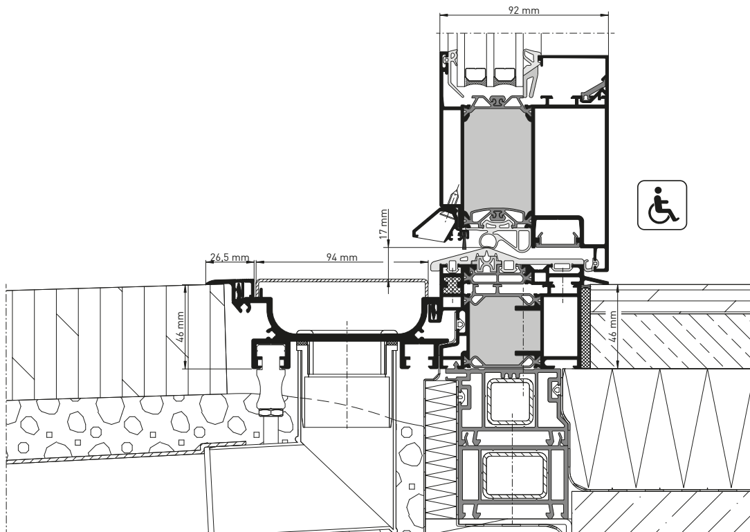
heroyal D 92 UD mit heroyal DS, Schnittdarstellung
