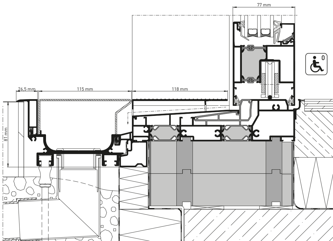
heroal S 77 SL mit heroal DS, barrierefrei nach DIN 18040, Schnittdarstellung
