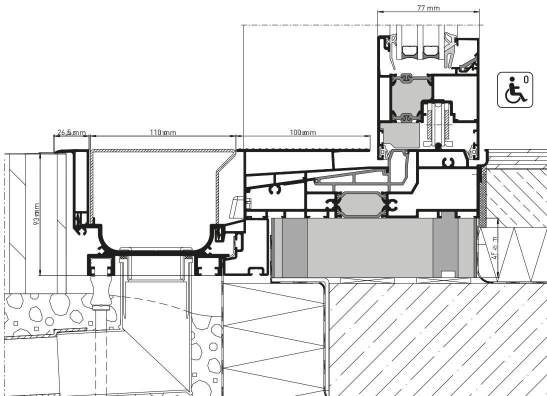
heroal S 77 mit heroal DS, barrierefrei nach DIN 18040, Schnittdarstellung
