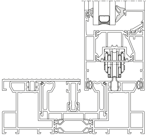
heroal S 65 mit Nullbarriere-Schwelle, ohne Zusatz-Dämmung und mit Standard-Dichtungen, Schnittdarstellung
