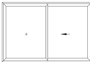
Beschlagschema A (rechts): 1 Schiebeflügel, 1 Festflügel
