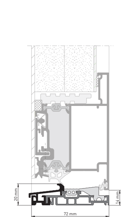
Durchlaufende Schwelle 2-teilig
