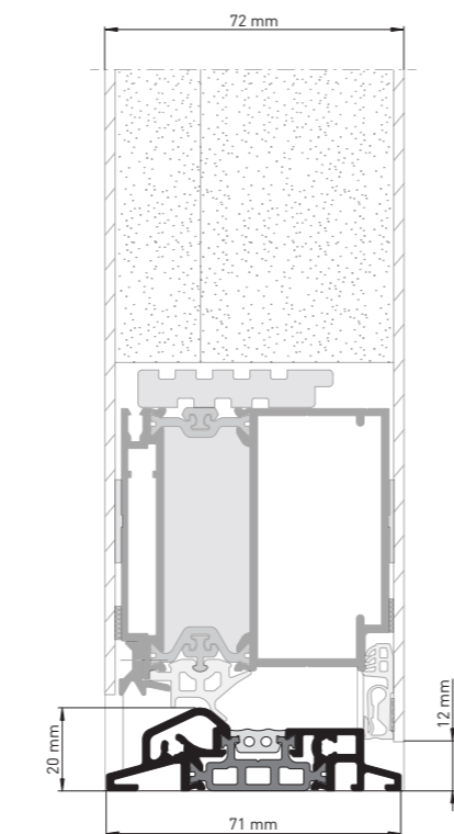
Schwelle mit Anschlagdichtung
