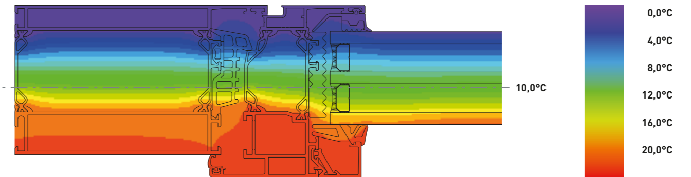
Isothermenverlauf nach U_f EN ISO 10077-2
