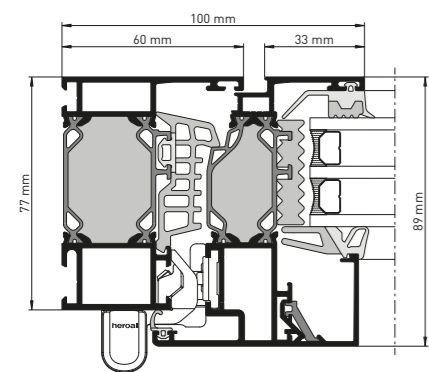
heroal W 77 mit Beschlagsystem heroal WF 100
