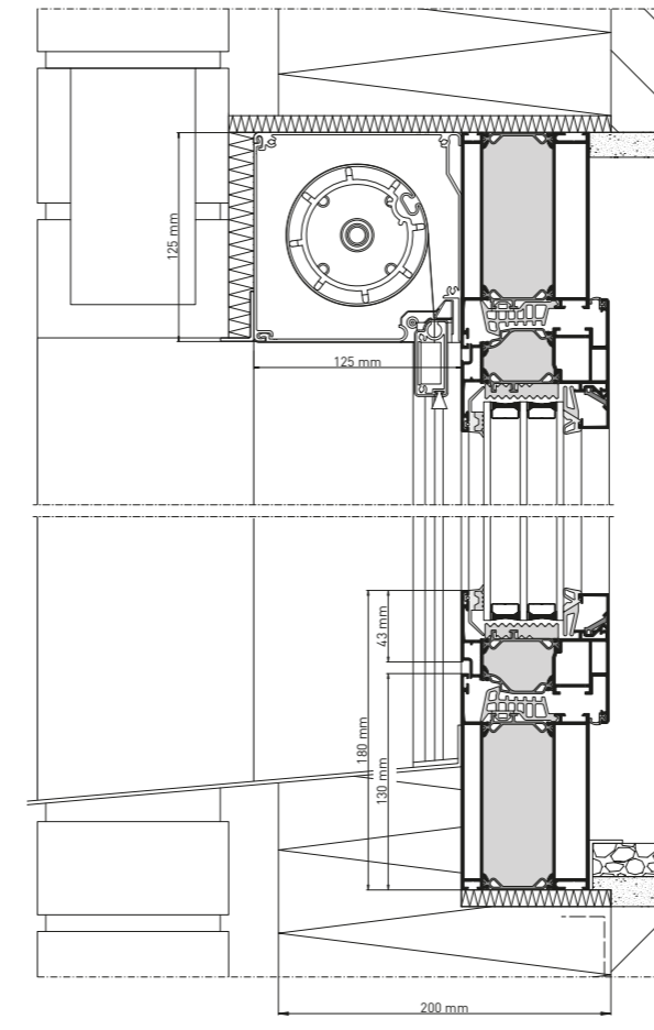
heroal W 77 PH mit Sonnenschutzsystem VS Z
