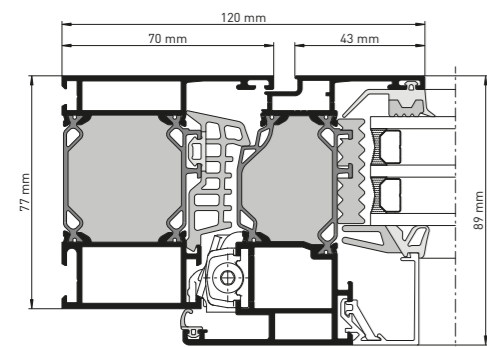
heroal W 77 mit Beschlagsystem heroal WF 100 i
