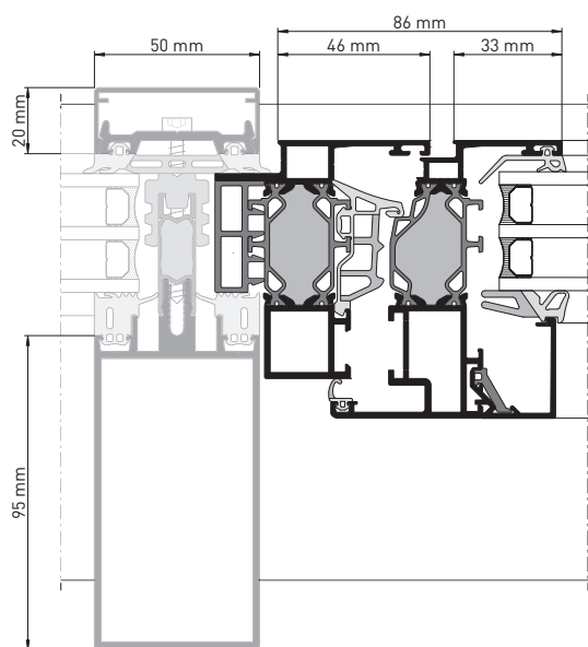
heroal W 72 als Einsetzelement im Fassadensystem heroal C 50
