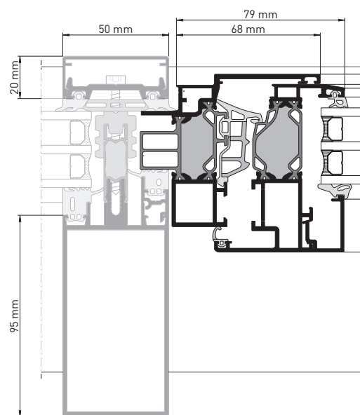
heroal W 72 i (Innenverglasung) als Einsetzelement im Fassadensystem heroal C 50
