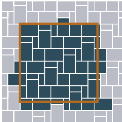
Römischer Verband
