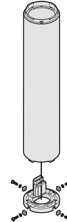
Standrohr 840 S
