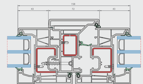
Horizontalschnitt
