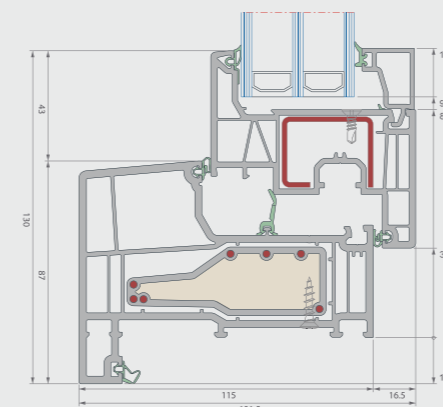
Vertikalschnitt
