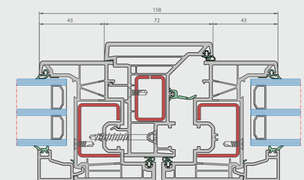
Horizontalschnitt
