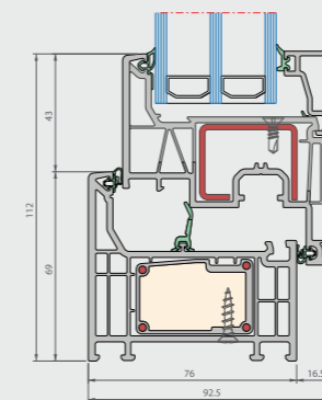
Vertikalschnitt
