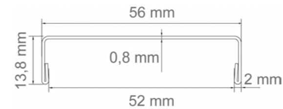
Edelstahlprofil 5 cm
