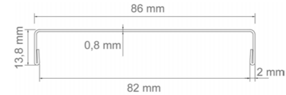
Edelstahlprofil 8 cm
