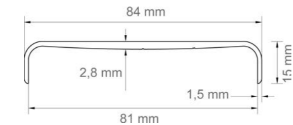
Aluminiumprofil
