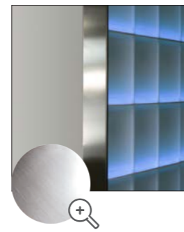
Edelstahl gebürstet für 8 cm Glasbausteine
