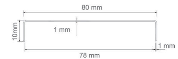
Edelstahlprofil 8 cm - ohne Gehrungsschnitt
