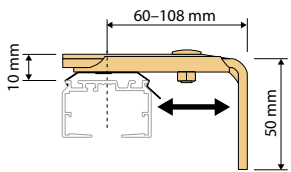
Montagefläche: 20 x 50 mm
