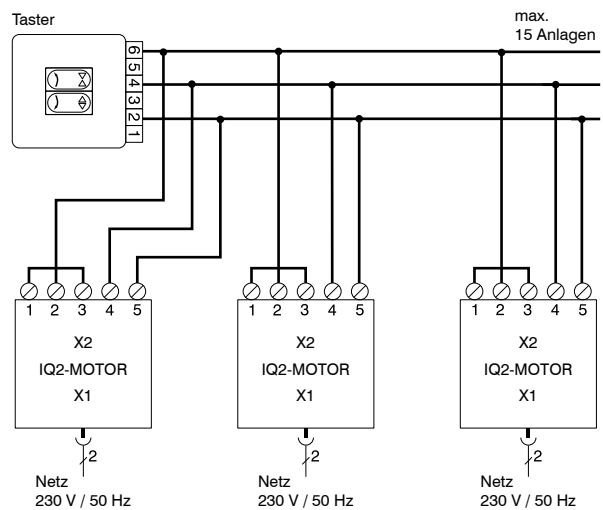
Anschlussplan
