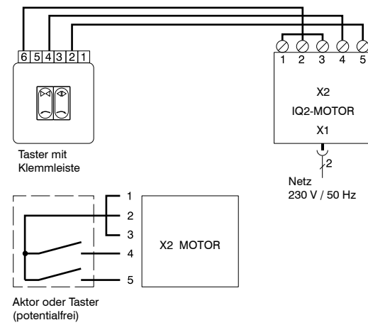
Anschlussplan
