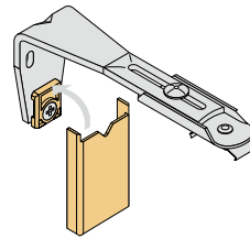
Abdeckkappe »groß« für Wandwinkel 108-156 mm für Wandwinkel 156-204 mm
