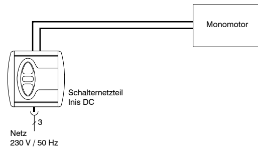
Anschlussplan
