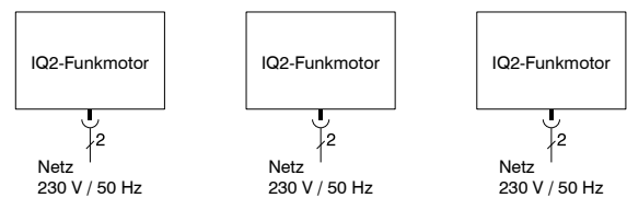
Anschlussplan
