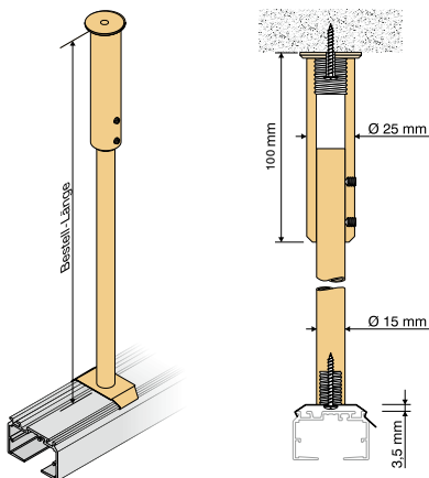
Abhänger mit Halteclip Bestellhinweis: Bitte Art.-Nummer und Bestelllänge angeben
