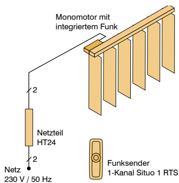
Prinzipschaltbild
