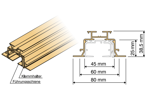
Einbauprofil (Klemmhalter gesondert bestellen)
