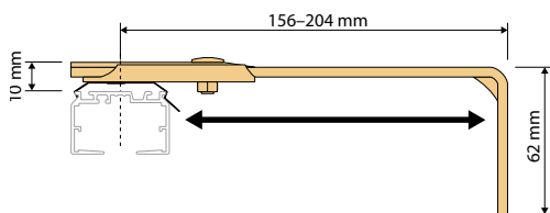
Montagefläche: 35 x 62 mm
