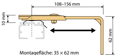
Montagefläche: 35 x 62 mm
