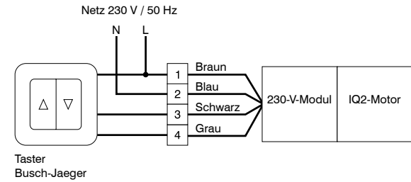
Anschlussplan
