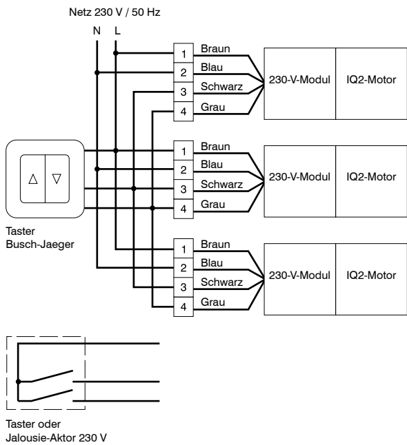
Anschlussplan
