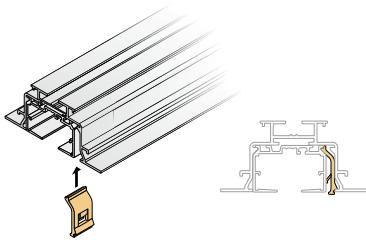
Klemmhalter
