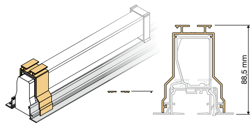
Motorhalter für Einbauprofil für verdeckten Einbau der Führungsschiene mit obenliegendem Motor, Einbauprofil muss für Motor und Zusatzmodule ausgeklinkt werden
