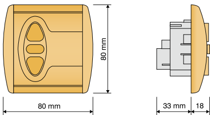
Schalternetzteil Inis DC max. 2 Monomotoren
