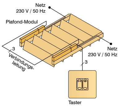
Prinzipschaltbild
