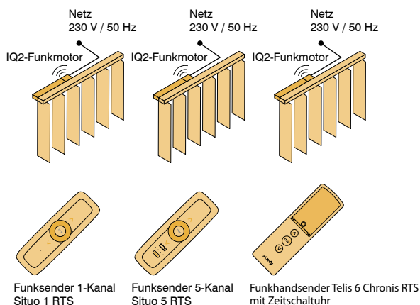
Prinzipschaltbild
