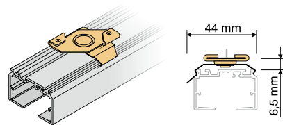
Schnellmontageclip mit Halteclip gekröpft für T-Profil 24–26 mm
