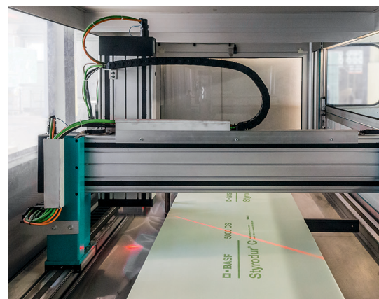
Vermessungsroboter
