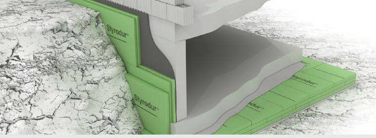
Perimeterdämmung
