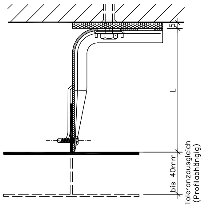
TOLERANZAUSGLEICH
