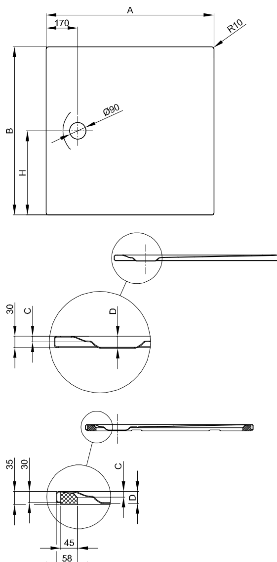
Darstellung mit vormontiertem Minimum-Wannenträger (T1).
