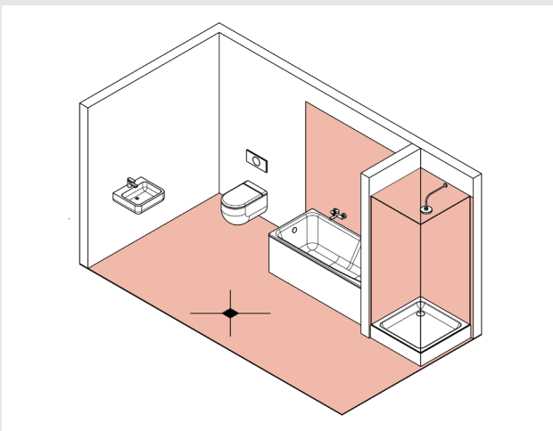
6. Häusliches Bad mit Badewanne, ohne Brause und mit Duschtasse mit Duschatrennung: Bodenablauf im Raum
