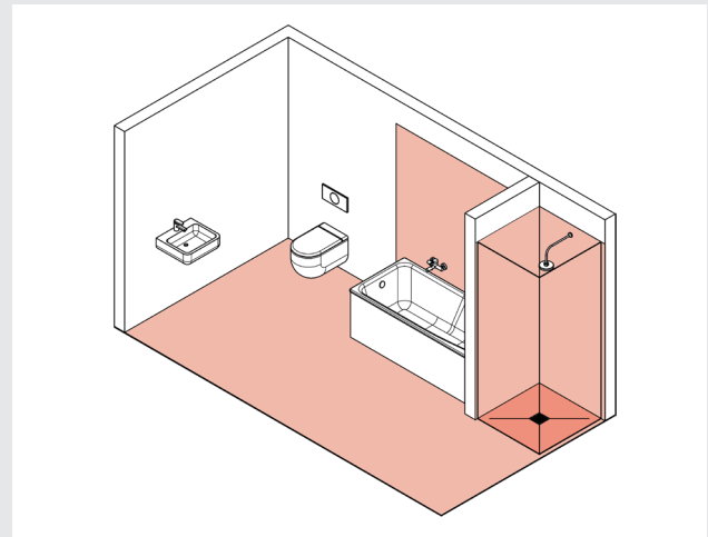
5. Häusliches Bad mit Badewanne, ohne Brause und mit bodengleicher Dusche mit Duschatrennung
