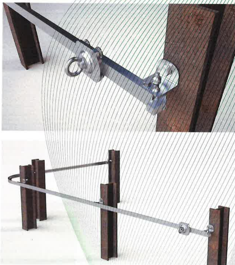
Bilder 1 - 2: Anschlageinrichtung, Typ: ABS RailTrax (Montagebeispiel)
