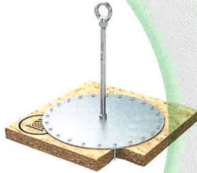
Bild 16: Anschlageinrichtung, Typ: ABS-Lock® X-H-24
