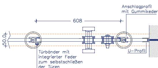
Horizontalschnitt
