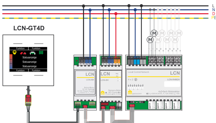
Zentrale Rollladensteuerung (mit LCN-GT4D)
