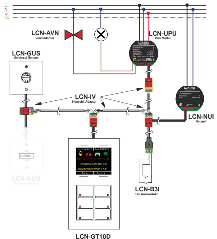
Abb.) Beispiel für mehrere Sensoren am gleichen Modul:
