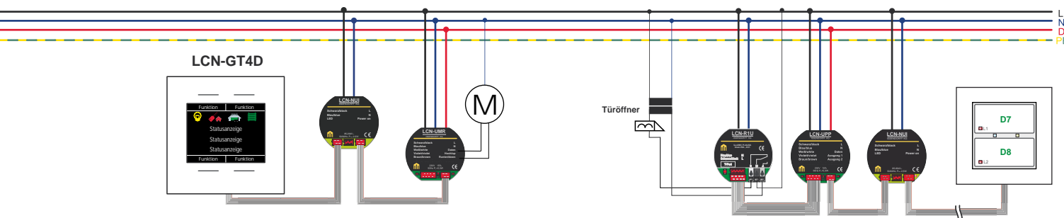
Einfache Rollladensteuerung (mit LCN-GT4D)
