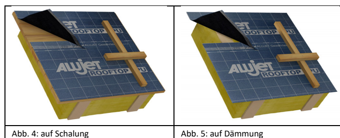
Abb. 4: auf Schalung
