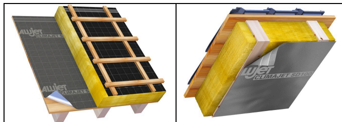
Abb. 3: Einsatz unter Aufdachdämmung
