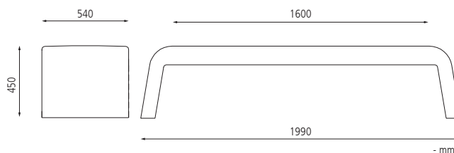
▲ Sitzbank ALBA aus UTC®-Beton, in dunkelgrau
