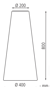
▲ Poller KONE aus Beton, in Granitoptik weiß
