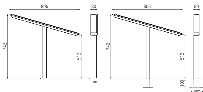
Anlehnbügel EGER zum Aufdübeln bei -100 mm, in RAL 6027 lichtgrün
