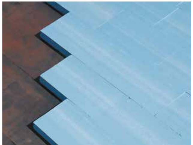
Abb. 17: Umkehrdach auf bituminöser Abdichtung
