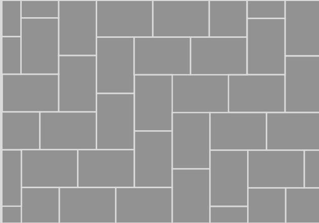
VERLEGEMUSTER FISCHGRÄTVERBAND ca. 33 Stck. // 21 x 14 x 8 cm/m 2
