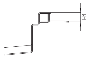
HF Haftflansch 1)
