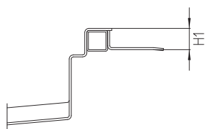
AF Anarbeitungsflansch 1)
