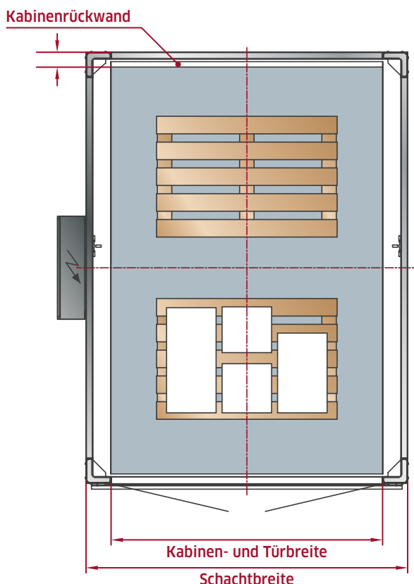
EINSEITIGE BELADUNG
