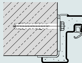
Schweißmontage mit Schiebeanke (Sichtmauerwerk)
