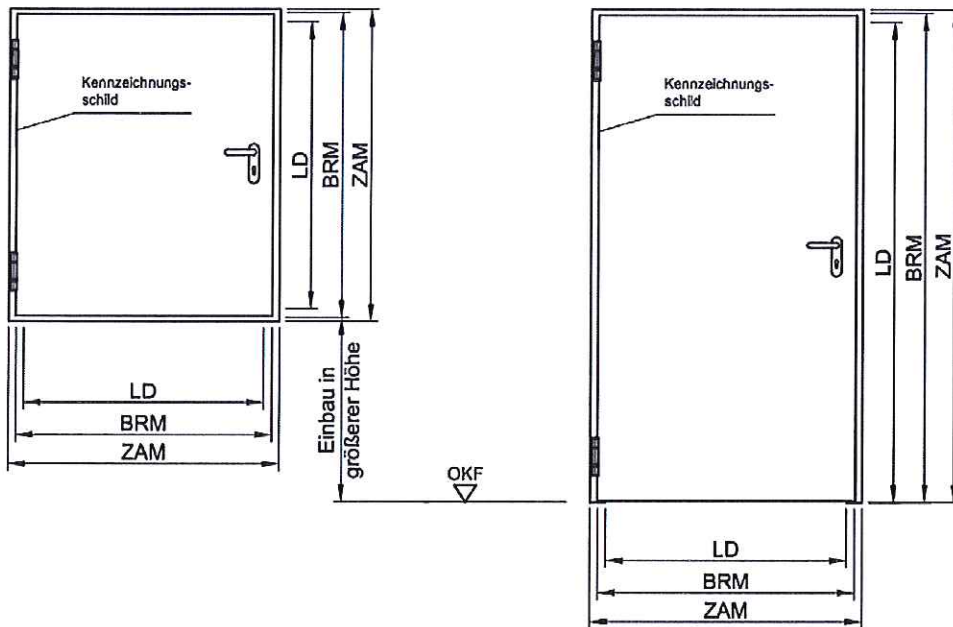
Dargestellt: Gangflügel DIN links, Gangflügel DIN rechts spiegelbildlich
