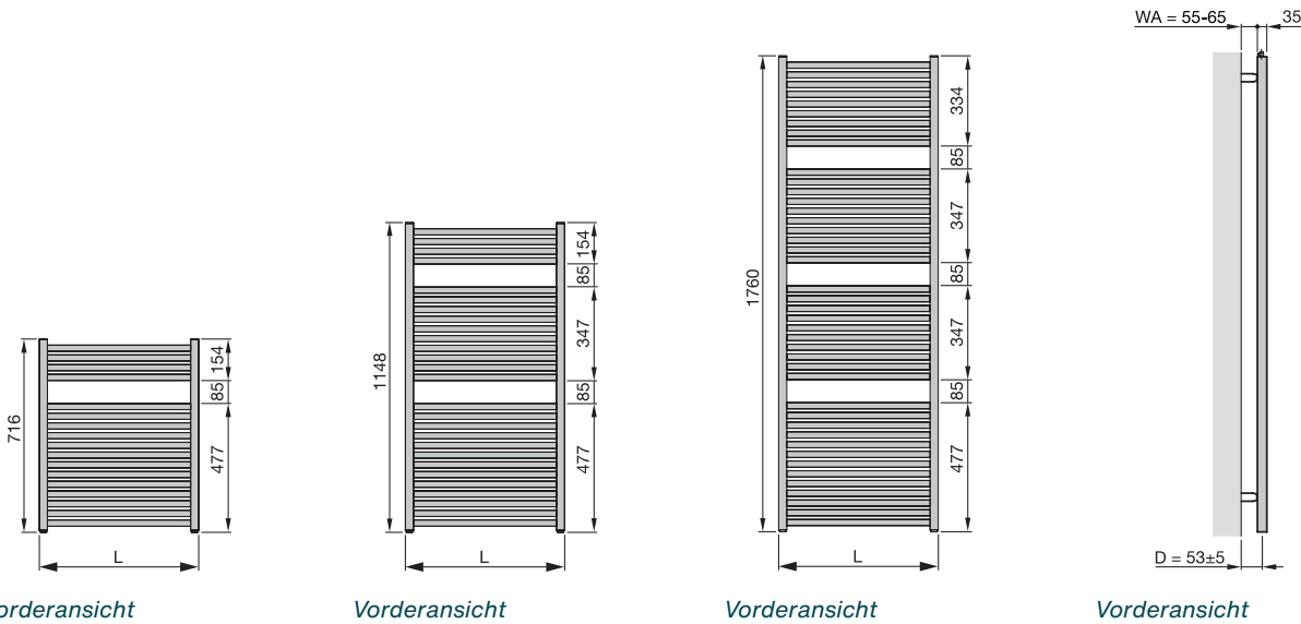
Vorderansicht
