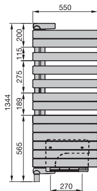
Vorderansicht, Ausführung rechts
