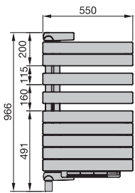
Vorderansicht, Ausführung rechts
