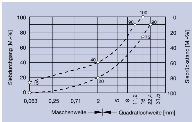
Bild 5: Sieblinienbereiche für HGDI/HGTD 0/16 mm und 0/22 mm entsprechend ZTV LW
