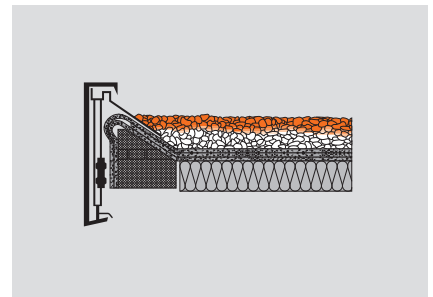
Mit PCI Stabiflex verfestigte Kiesschüttung. PCI Stabiflex fließt nicht auf die Dachhaut ab, sondern verfestigt die obere Schicht. Regenwasser kann ungehindert in das Kiesbett eindringen.
