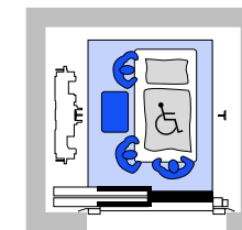
2.500 kg Kabine: 1.800 × 2.700 mm Türbreite: 1.400 mm Bett: 1.000 × 2.300 mm + Geräte
