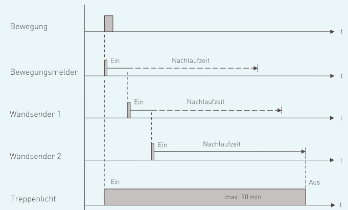
Funktionsprinzip Treppenlichtschaltung
