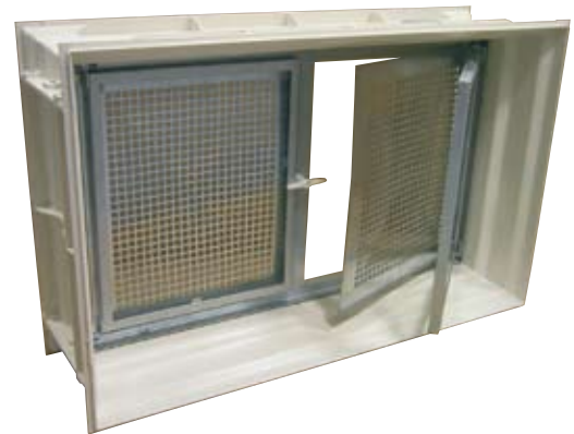
Zargenfenster Typ ZO mit Stahlkellerfenstereinsatz Typ SD 2
