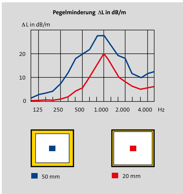
Pegelminderung schallabsorbierender Kanalauskleidungen
