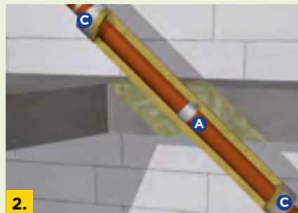
2. Schrägeinbau mit U Protect Roll 3.1 Alu1
