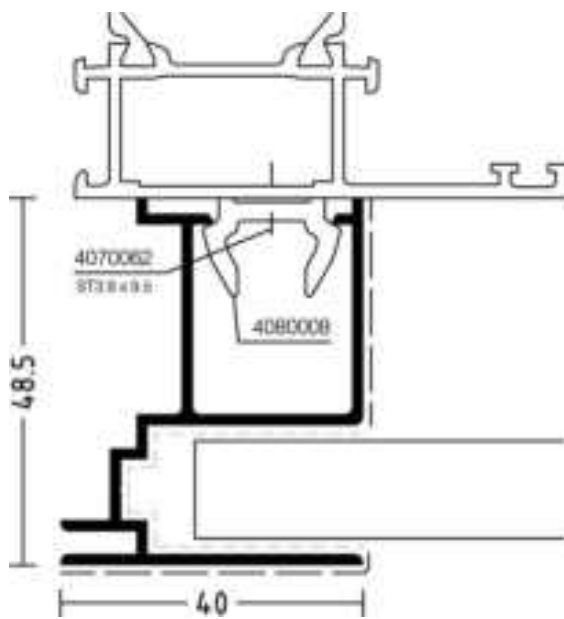
3091051 Führungsprofil Guide profile
