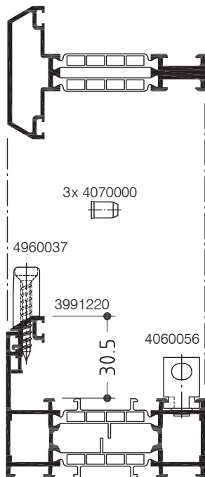
Sprosse / Blendrahmen mit Zusatzprofil Glazing bar / Frame with supplementary profile
