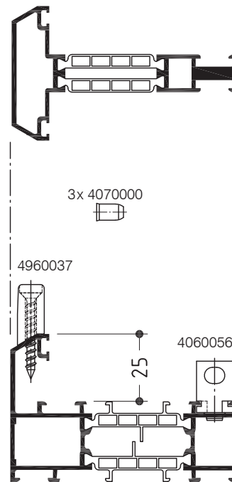
Sprosse / Blendrahmen Glazing bar / Frame
