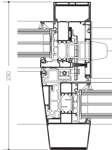
Mittelpfosten verstärkte Ausführung
