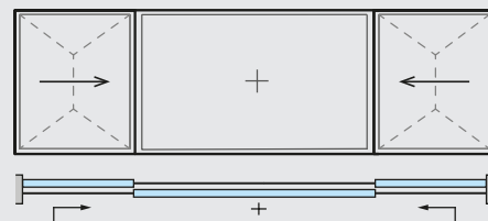
2 Schiebeflügel + 1 Festfeld
