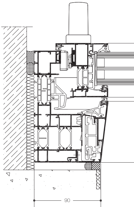
Horizontalschnitt – verdeckter Flügel
