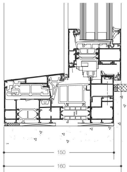
Vertikalschnitt – Öffnungsflügel, eingelassene Schwelle
