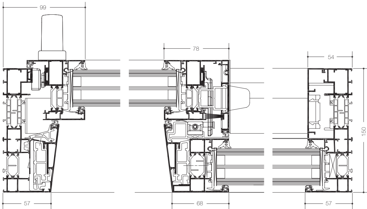
Horizontalschnitt 1 Schiebeflügel + Festfeld
