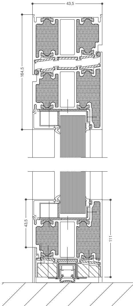
Anschlagtür, auswärts Spezialblendrahmen und Türflügelprofil umlaufend mit Absenktdichtung
