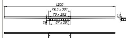
Duschrinne CeraWall Connect schwarz matt
