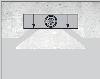
Betonkantenbruch
