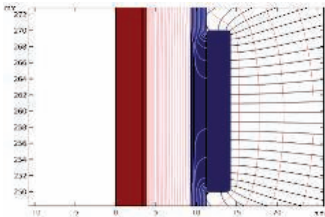
Felddiagramm einer isolierten Ableitung an der ersten Potentialausgleichsklemme während einer Typenprüfung zum Zeitpunkt t = 1,2 \mu\text{s} der angelegten Impulsspannung 1,2/50.
