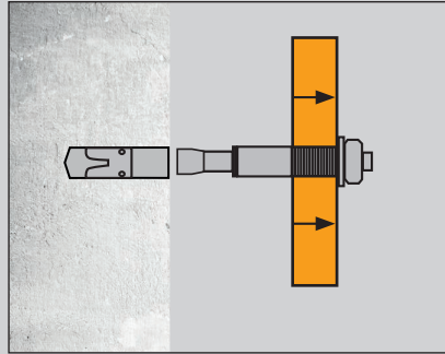
Durchziehen
