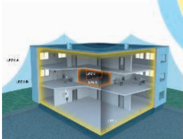
Schutzprinzip nach dem Blitzschutzonenkonzept
