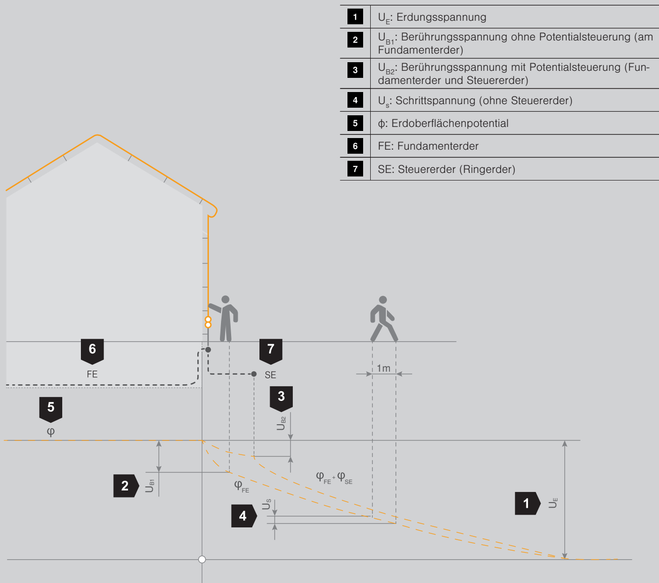
Erdoberflächenpotential und Spannungen beim stromdurchflossenen Fundamenterder FE und Steuererder SE
