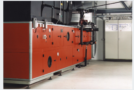
Im Keller aufgestellte RLT-Anlage
