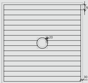
Fundo Primo/Ligno Plus 1.200 × 1.200 mm 2,7 × wedi 610
