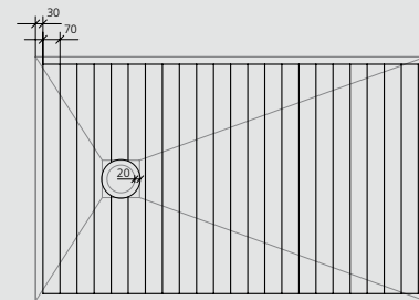
Fundo Primo/Ligno Plus/ Plano 1.600 × 1.000 mm 3 × wedi 610
