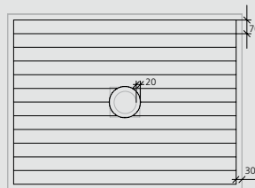
Fundo Primo/Plano/Integro 1.200 × 900 mm 2 × wedi 610
