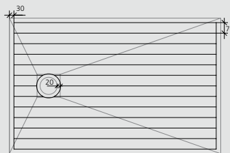
Fundo Primo/Ligno Plus 1.400 × 900 mm 2,4 × wedi 610
