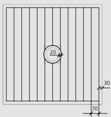
Fundo Primo/Ligno Plus/ Plano/Integro 900 × 900 mm 1,7 × wedi 610
