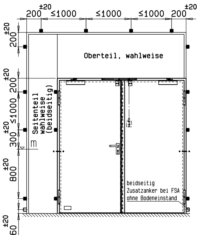
zweiflügeliger FSA als Tür
